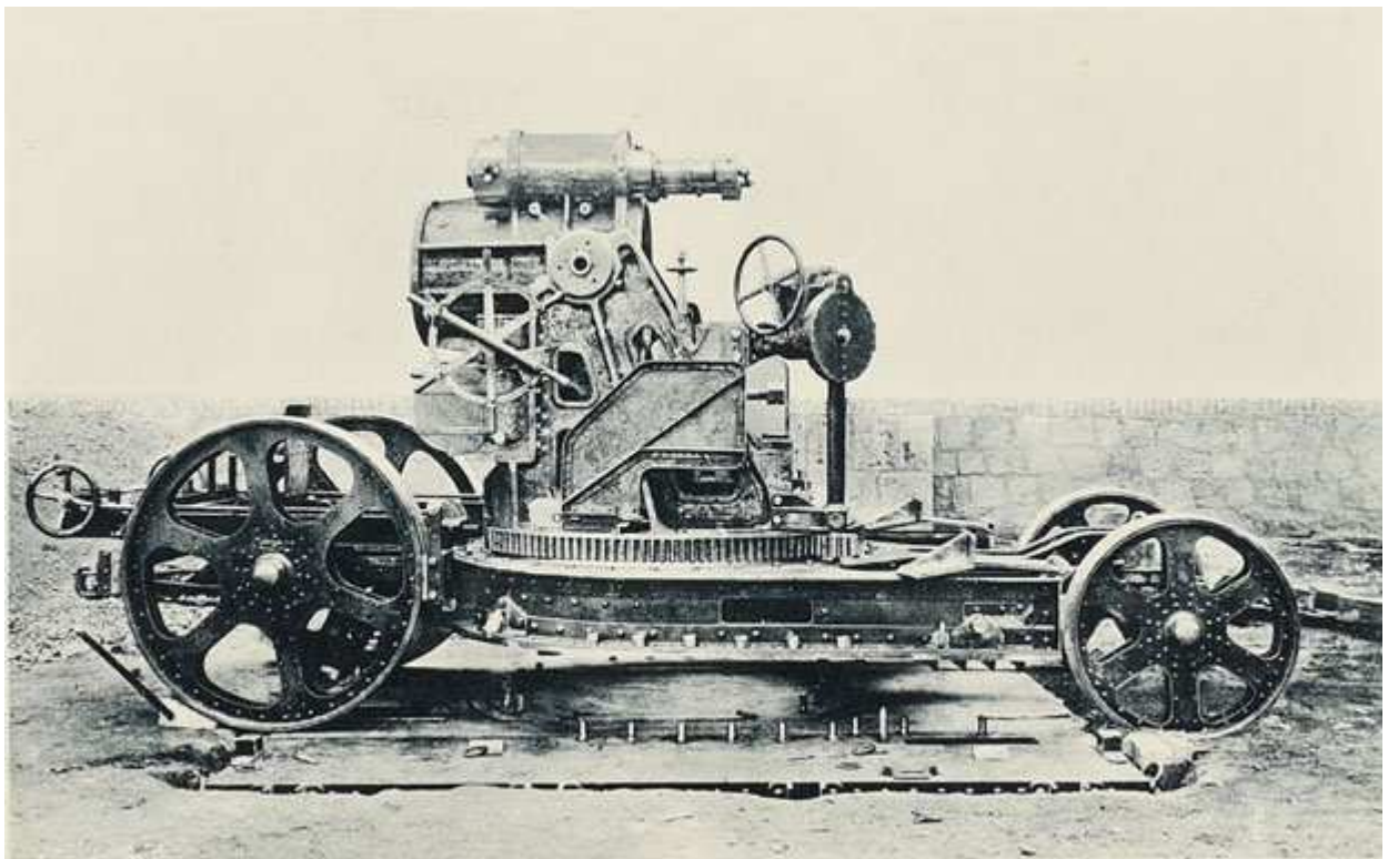
30.5 cm Belagerungsmörser M 11. Lafettenwagen.
