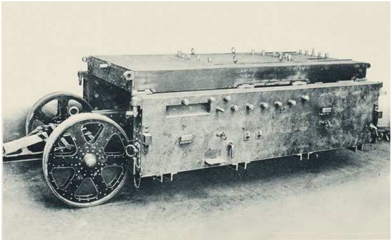
30.5 cm Belagerungsmörser M 11. Bettungswagen.
