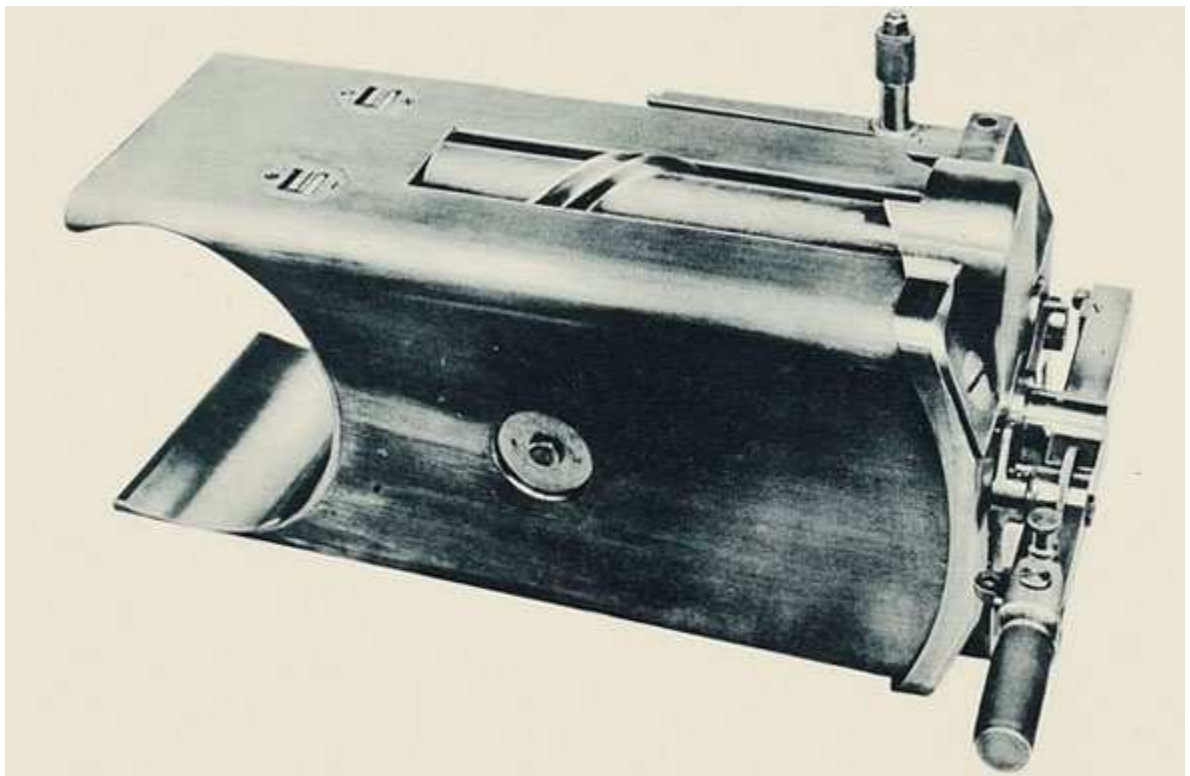
30.5 cm Belagerungsmörser M 11. Verschluß. Ansicht von rückwärts.
