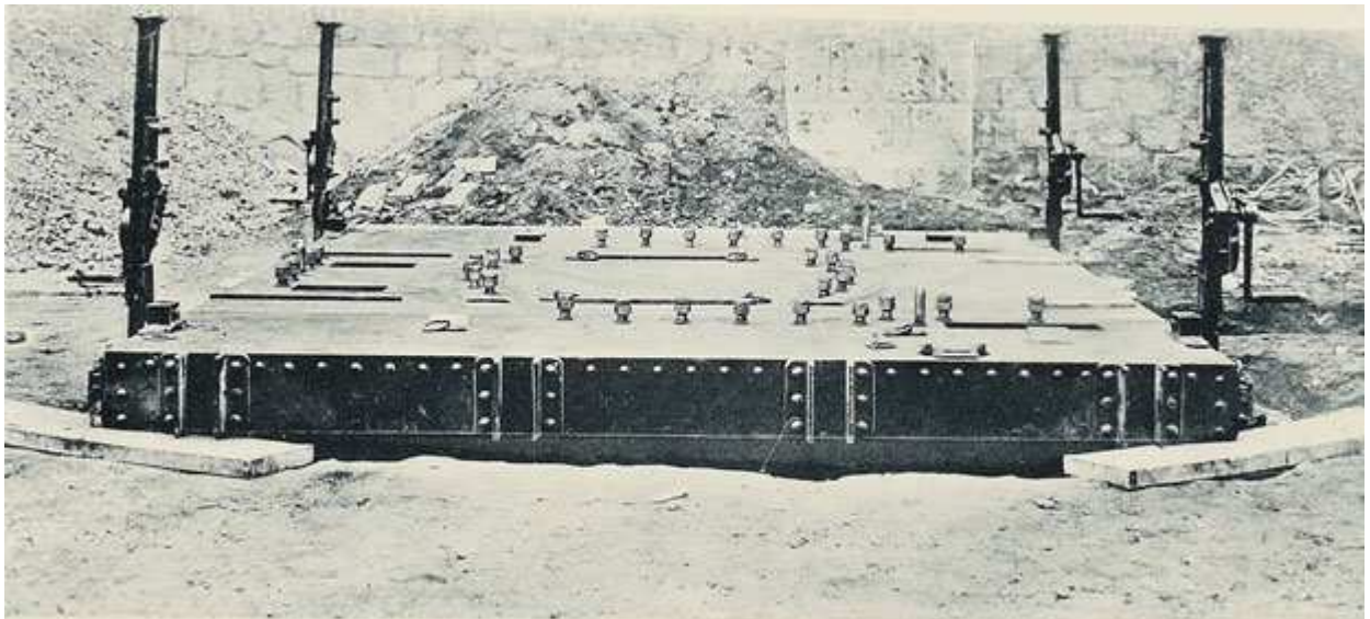
30.5 cm Belagerungsmörser M 11. Legen der Bettung.
