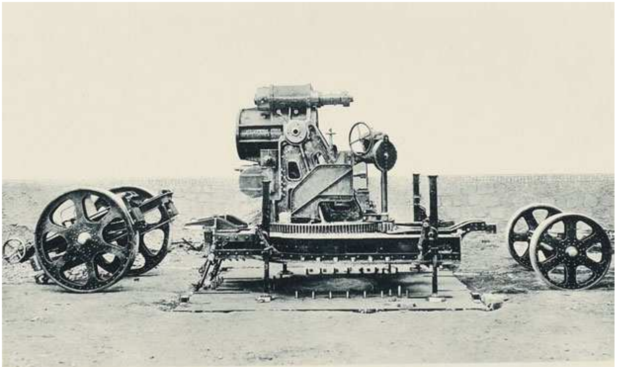
30.5 cm Belagerungsmörser M 11. Abprotzen der Lafette.
